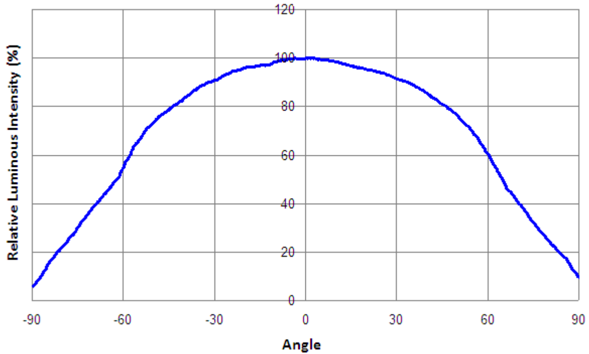
N5050U-UNF4 (beam angle 65°)
