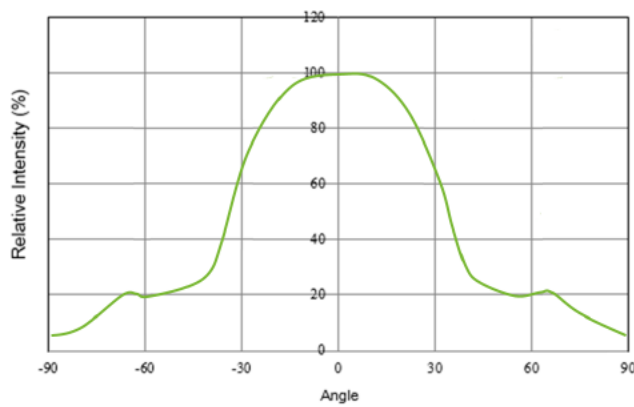
N3535X-INFx (beam angle 65°)
