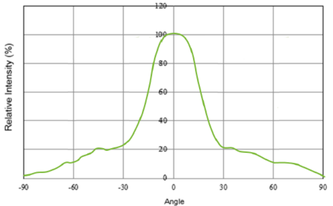
N3535X-INSx (beam angle 30°)
