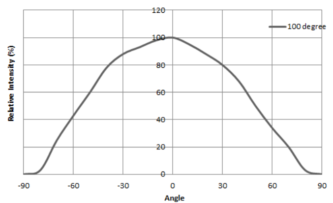
N3535X-JNAx series (beam angle 100°)
